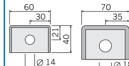
Baugröße / Size 040 - 050 071 - 080
