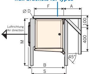
Wandkonsolen für Typen 040.2, 045.2, 050.2 wall brackets for types
