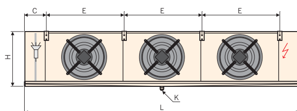
Wandkonsolen für Typen 040.2, 045.2, 050.2 wall brackets for types
