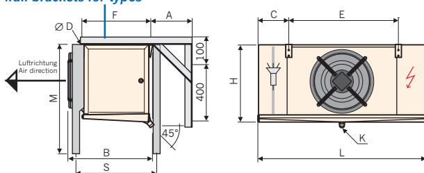
Wandkonsolen für Typen 040.2, 045.2, 050.2 wall brackets for types
