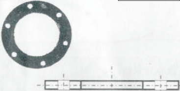
ZAPTIVKA BOJLERA KONČAR 6 OTVORA \phi 142/80 \times 3.5 ; VELIKI BOJLER
