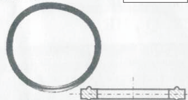
ZAPTIVKA BOJLERA MEBOŠ ORING \phi 114/90 \times 3.5
