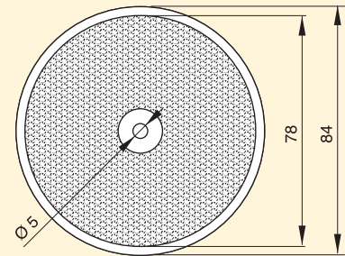
CTR6-RFL000015 Spessore 8,5 mm
