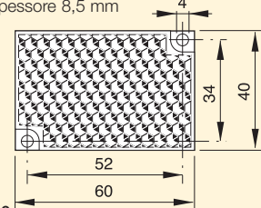
CTR6-RFL000015 Spessore 8,5 mm
