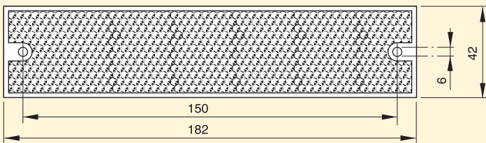
CTR8-RFL000017 Spessore 8 mm
