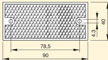
CTR2-RFL000013 Spessore 5 mm
