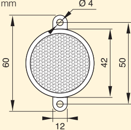
CTR1-RFL000012 ADESIVO Spessore 6 mm
