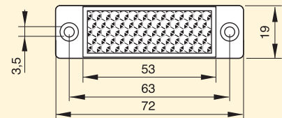
CTR10-RFL000018 Spessore 9,5 mm
