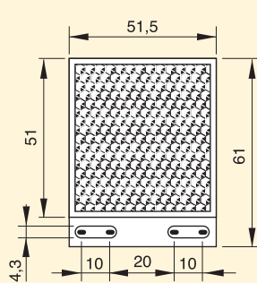
CTR8-RFL000017 Spessore 8 mm
