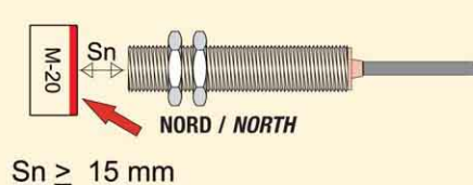
CHIUSURA CONTATTO CON IL NORD ACTIVATED BY THE NORTH POLARITY
