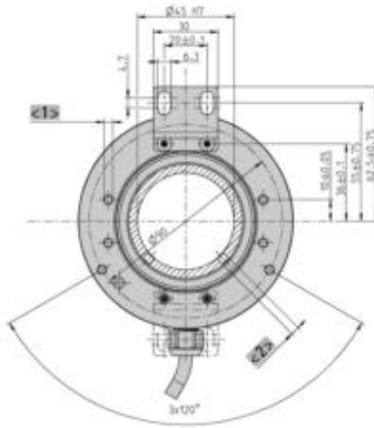
<2> M4 (2 x 90°)
