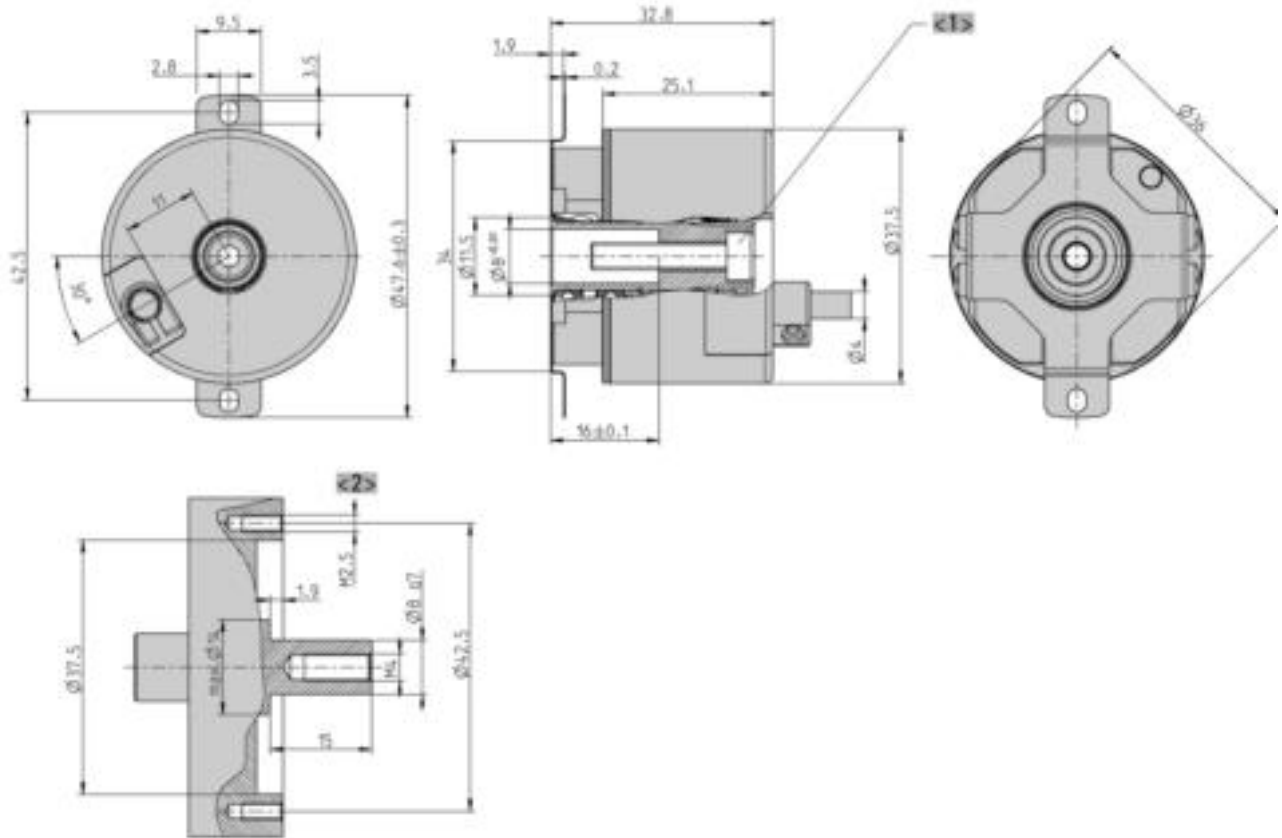
<1> ISO 4762 M4x20
