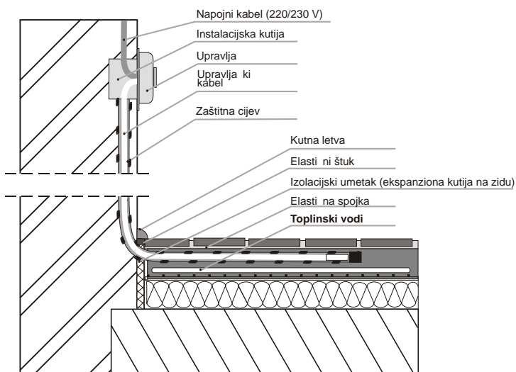
Slika 3b Temperaturni upravlja s podnim osjetnikom - instalacija
